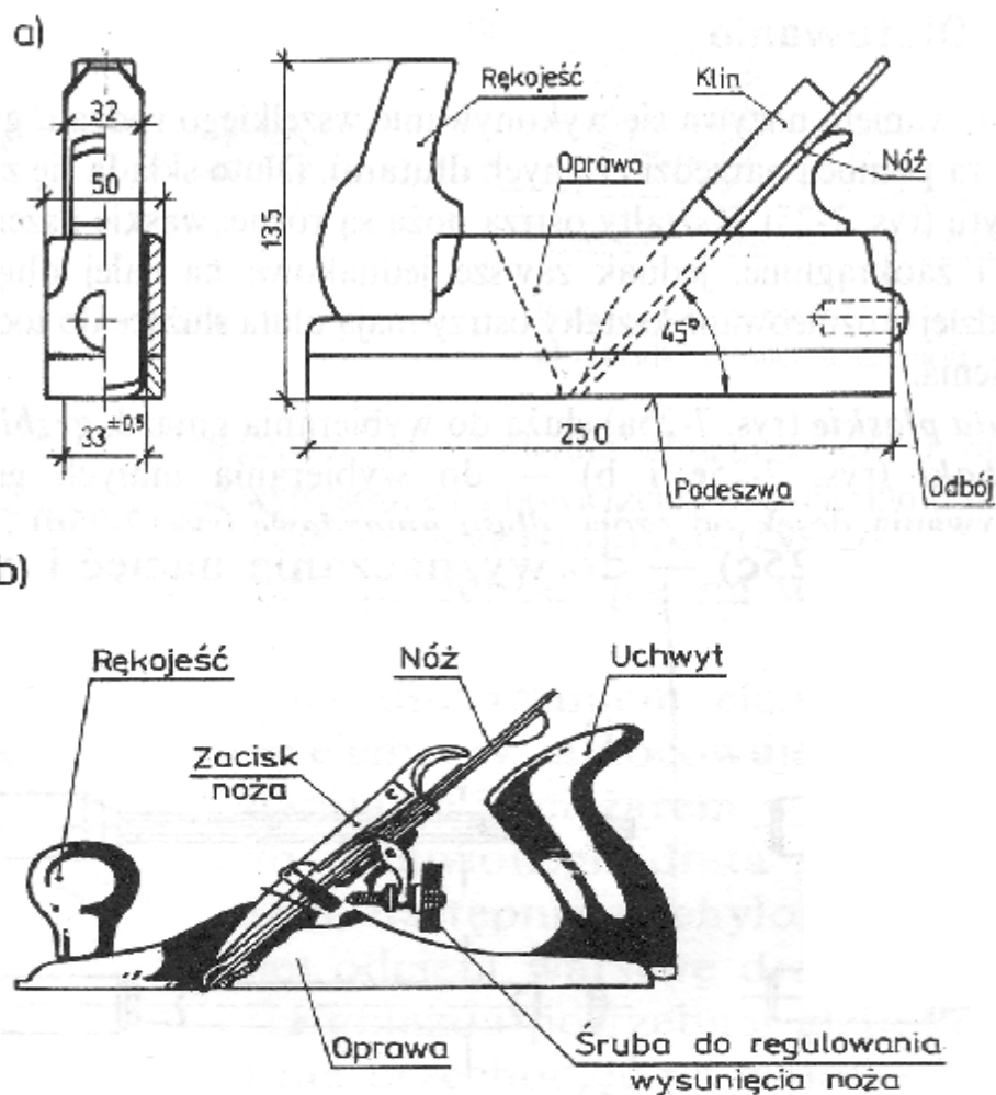
Rys. 14. Strugi: a) drewniane, b) metalowe [3, s. 123]
