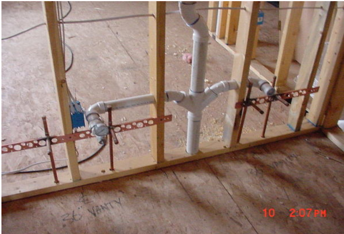
Montaż uchwyty pod armaturę
